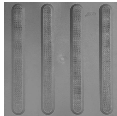
型號： HWS-003-G ( 方向導向地板 )
